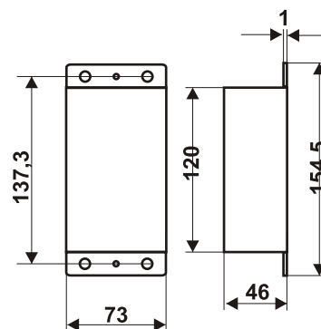
ΚΟΥΤΙ ΟΡΟΦΩΝ
