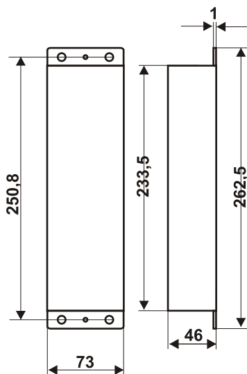
ΚΟΥΤΙ ΗΛΕΚΤΡΟΝΙΚΗΣ ΙΣΟΓΕΙΟΥ
